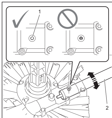
► 1. Trou 2. Tube
